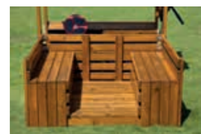
Sitzbänke hinten rear benches
